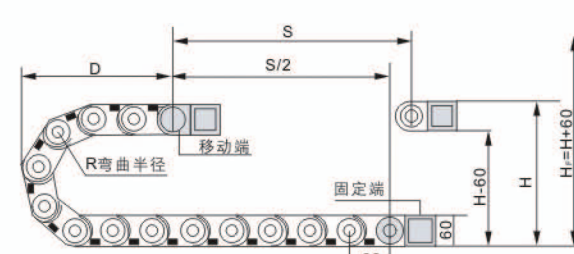
接头安装尺寸图
