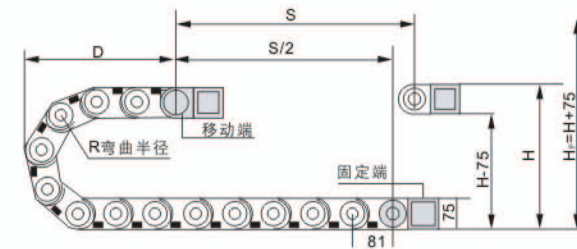
接头安装尺寸图
