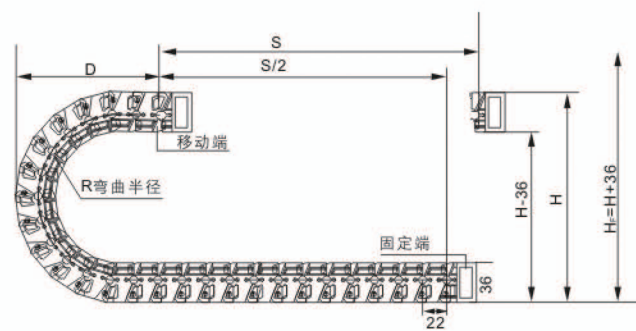
接头安装尺寸图
