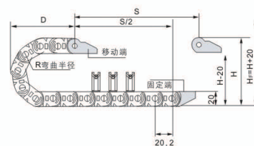
接头安装尺寸图
